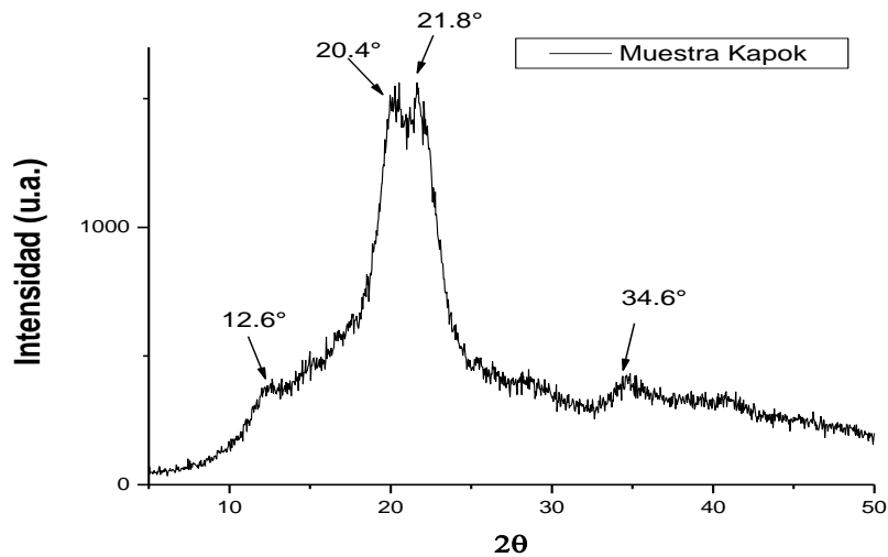
Figura 4. Diffractograma de la muestra de kapok
