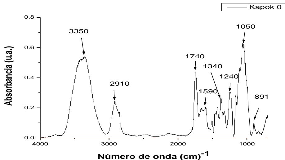
Figura 2. Interferograma de kapok ( Ceiba pentandra (L.) Gaertn)
