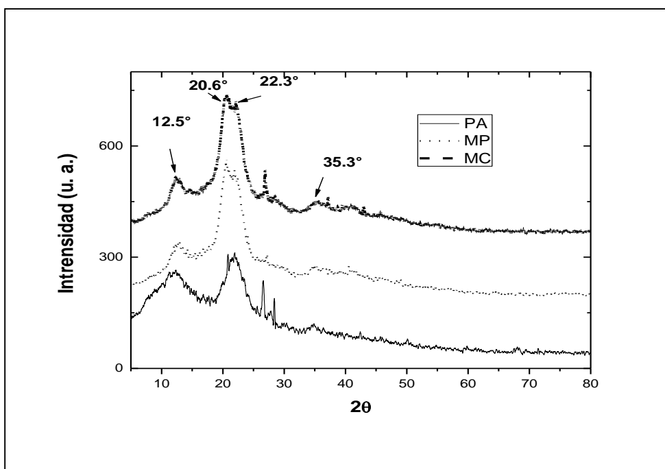
Figura 4. Difractogramas de las muestras de paja de caña (PA), celulosa extraída con el método de pulpeo en laboratorio (MP), celulosa extraída con el método casero (MC).
