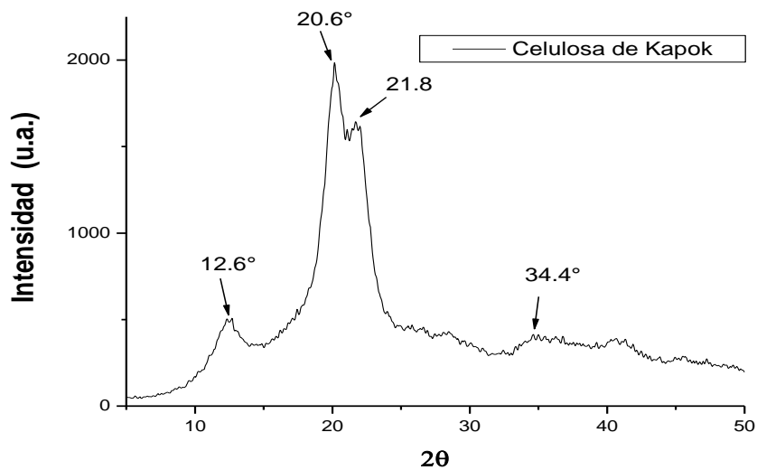
Figura 5. Diffractograma de la celulosa extraída
