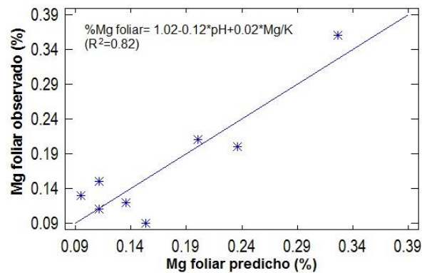
Figura 2. Validación cruzada de la absorción de Mg en hojas de maíz con la relación combinada pH-Mg/K
