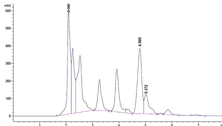
Figura 2. Cromatograma de extracción química convencional con sistema Soxhlet. Señal de esteviósido a 5.172 min (0.98 mg/ml) y señal de rebaudiósido “A” a 4.905 min (3.40 mg/ml).
